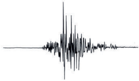
Il sismogramma del 6 maggio 1976, alle ore 21:00:12 (CEST)
